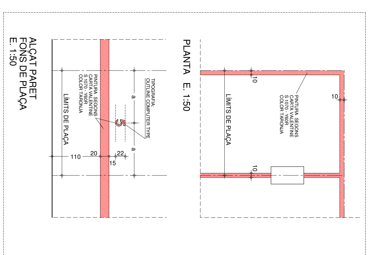
ESQUEMA PINTAT DE PLAÇA DE PARKING
