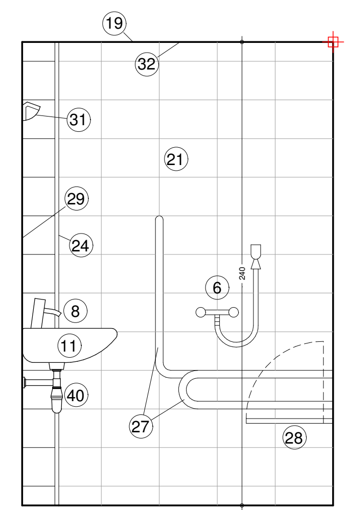
SECCIÓ 2-2'
