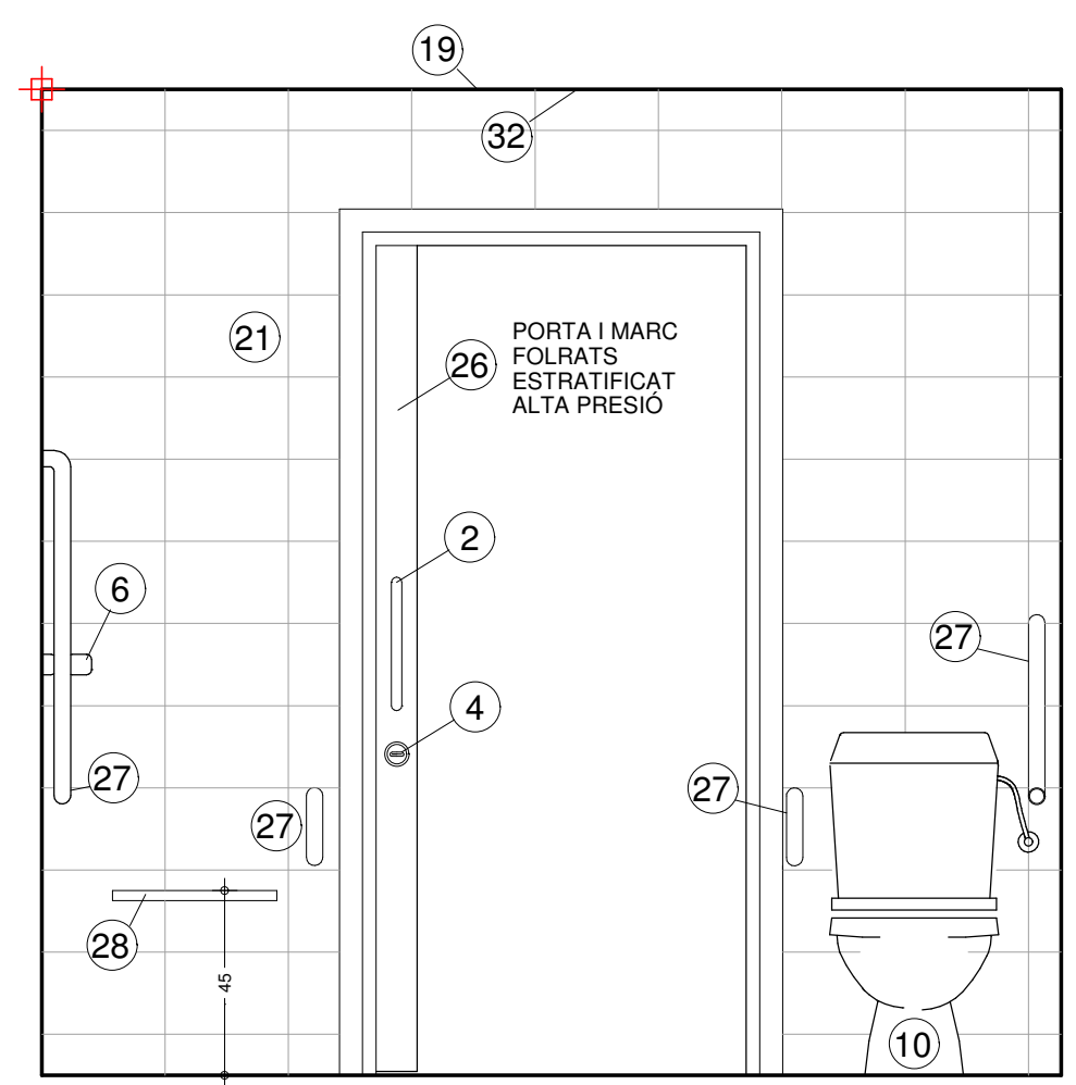
SECCIÓ 3-3'
