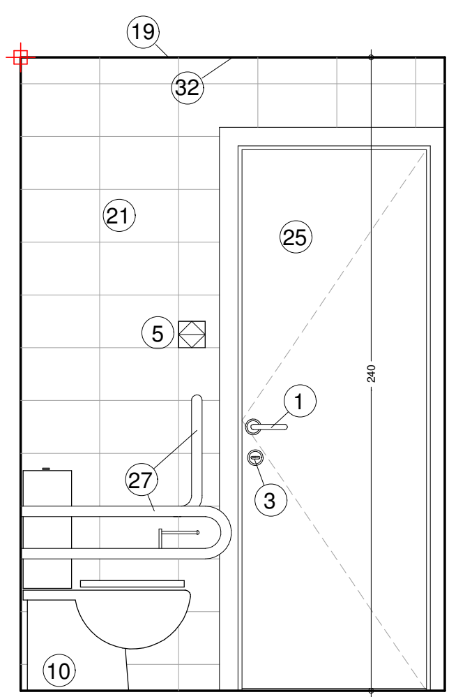
SECCIÓ 4-4'
