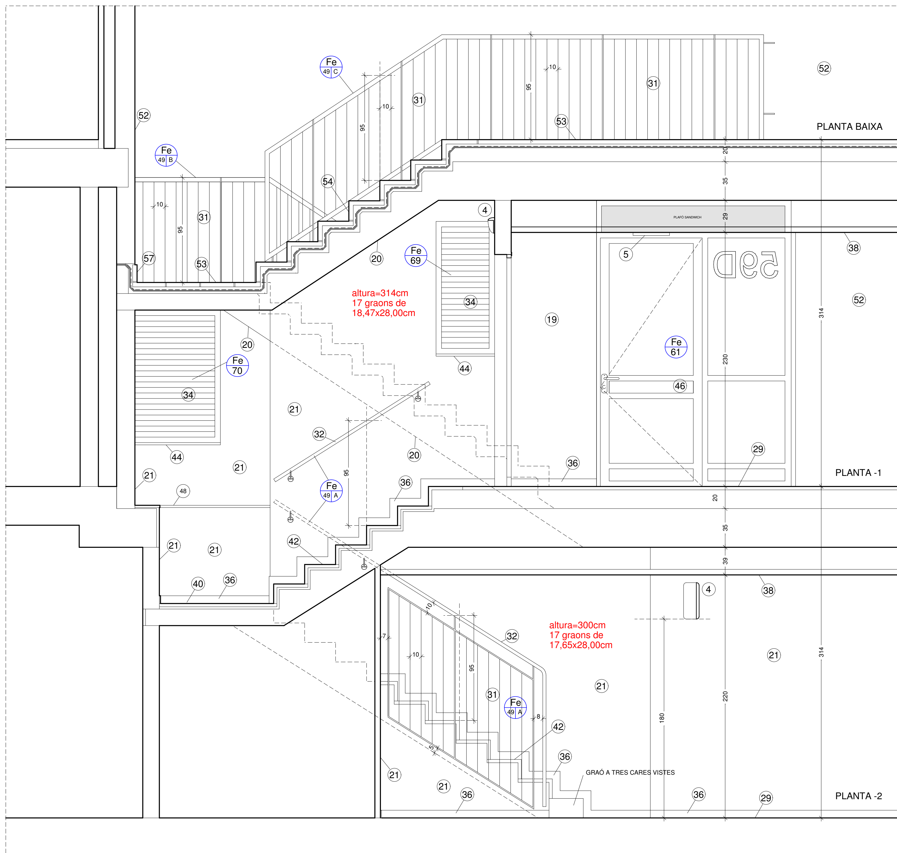
SECCIÓ A-A'
