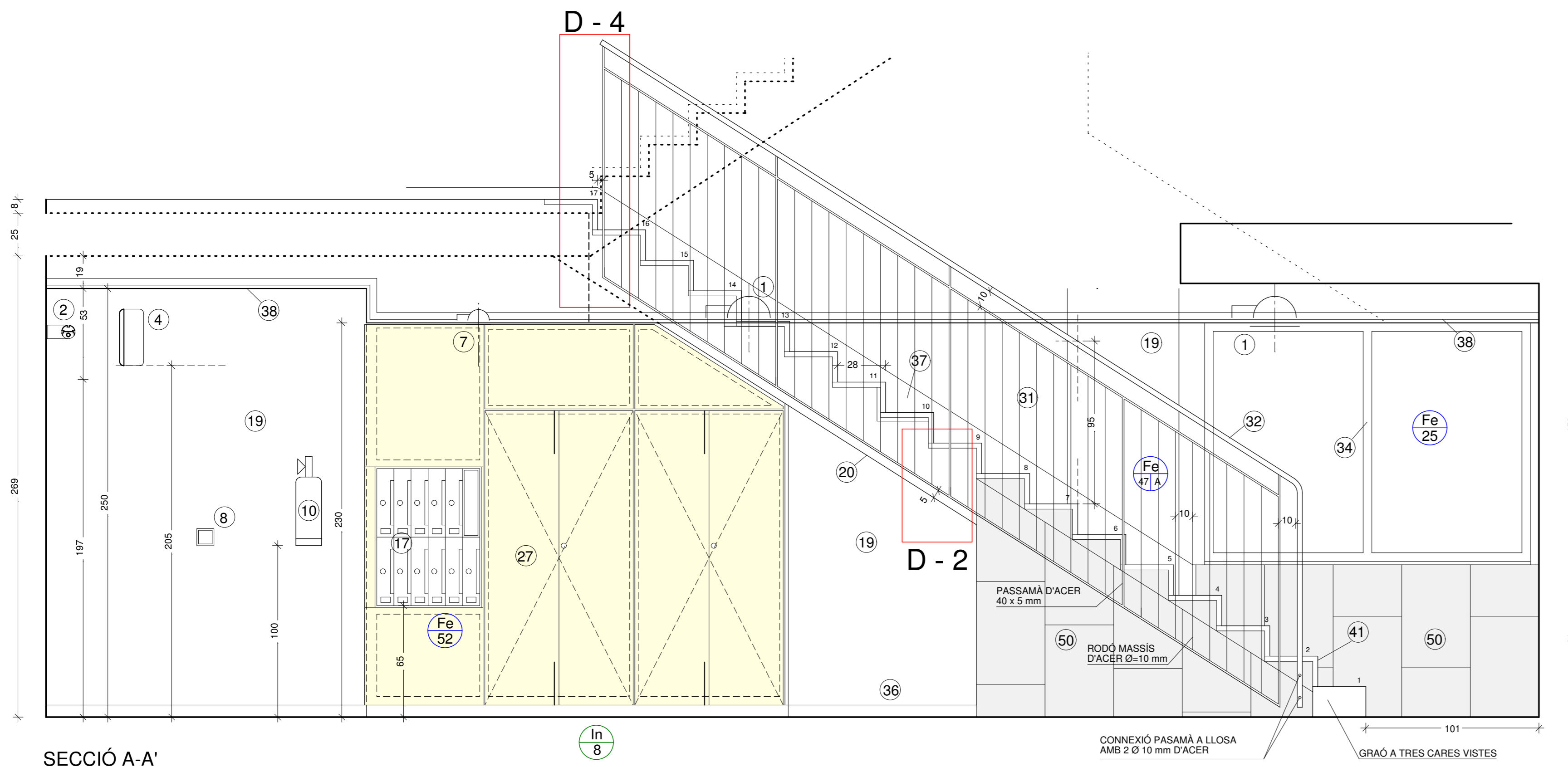
SECCIÓ A-A'
