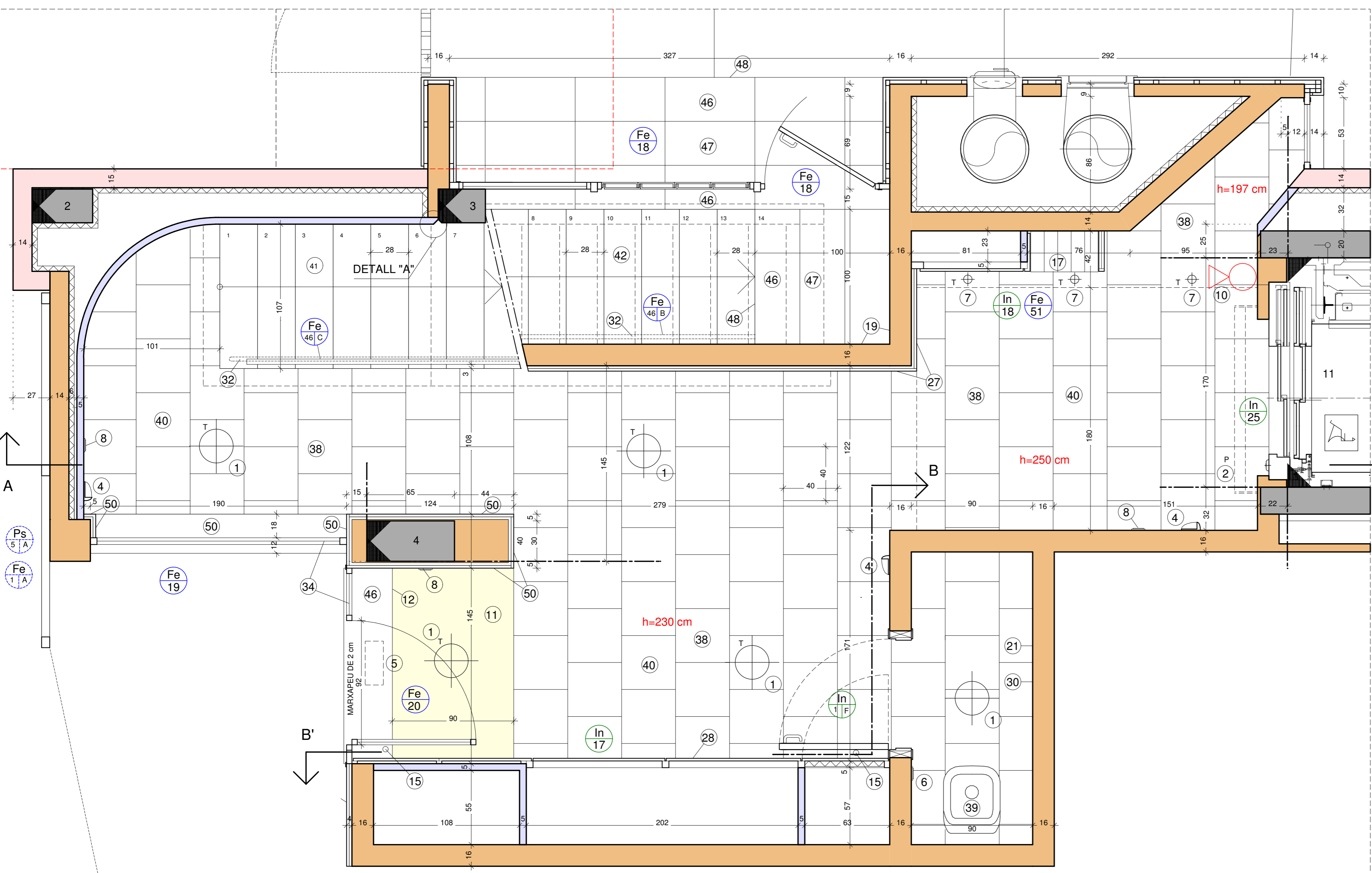
PLANTA BAIXA VESTÍBUL
