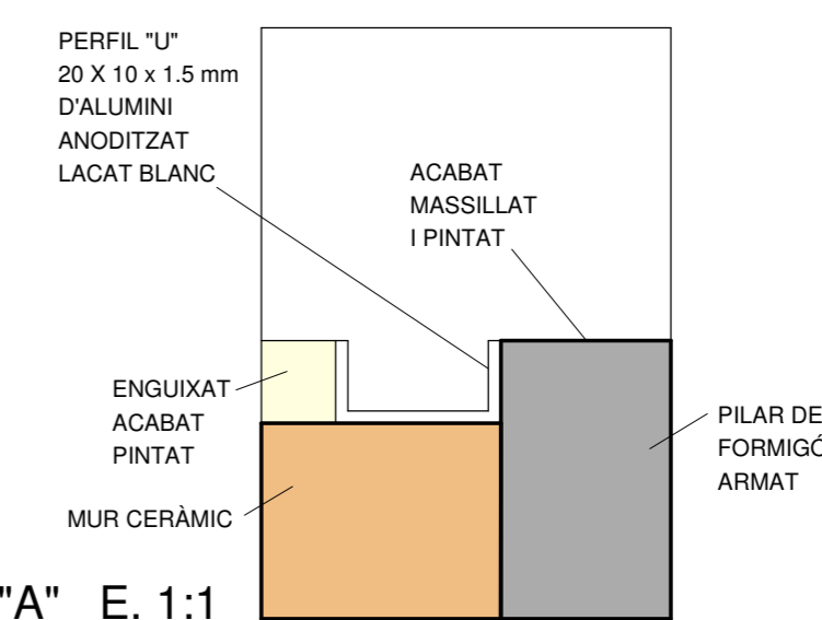
DETALL "A" E. 1:1
