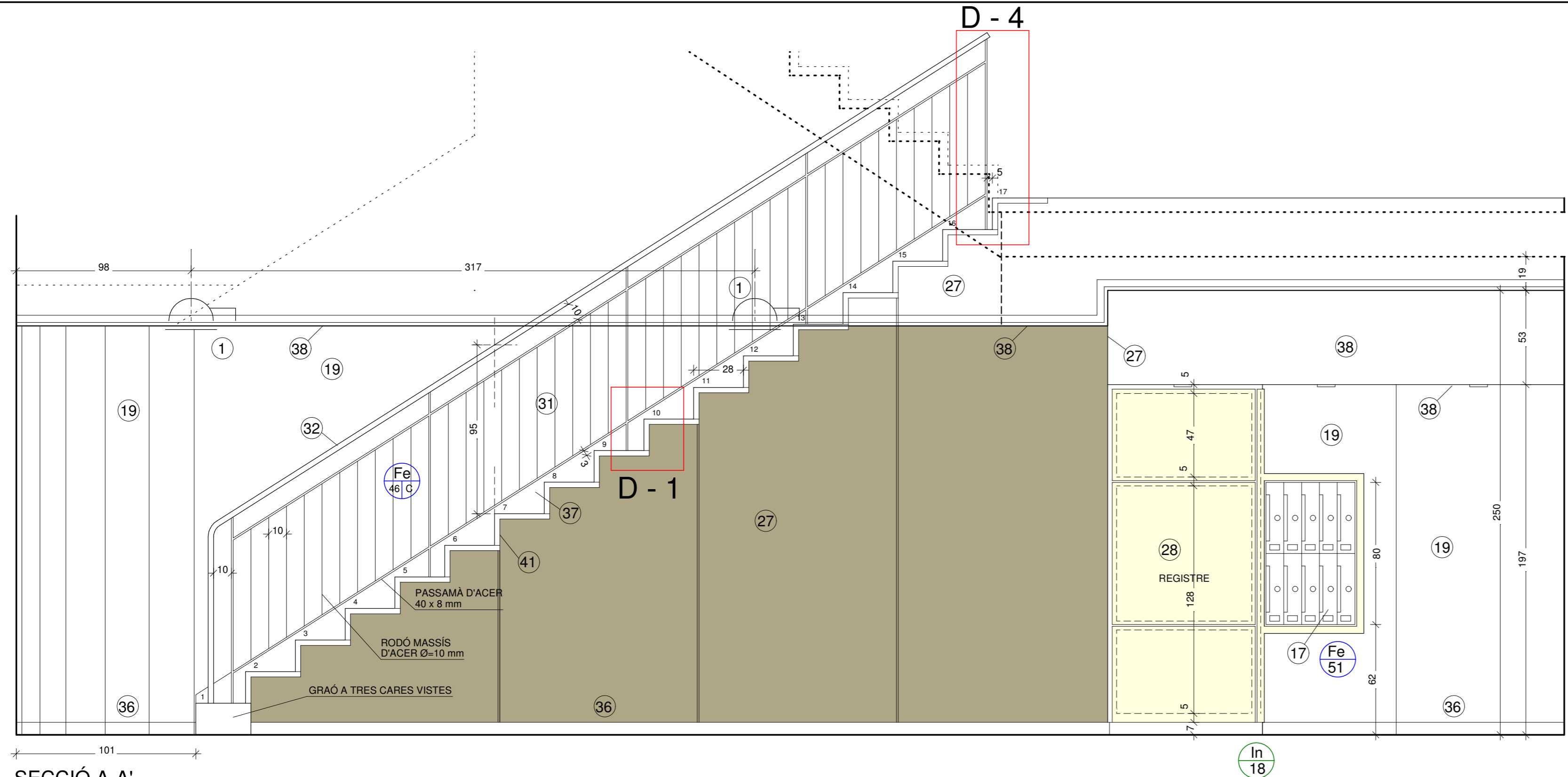
SECCIÓ A-A'
